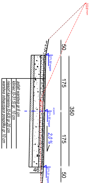
Przekrój 1-11 km 0+384,60
