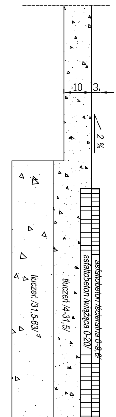
SCHEMAT NAWIERZCHNI JEZDNI WRAZ Z POBOCZEM
