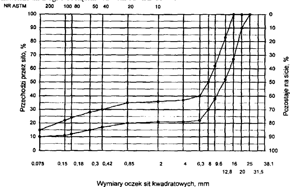
Rys. 1. Krzywe graniczne uziarnienia mieszanki mineralnej BA od 0 do 20 mm do warstwy scieralnej nawierzchni drogi o obciazeniu ruchem od KR3 do KR6
