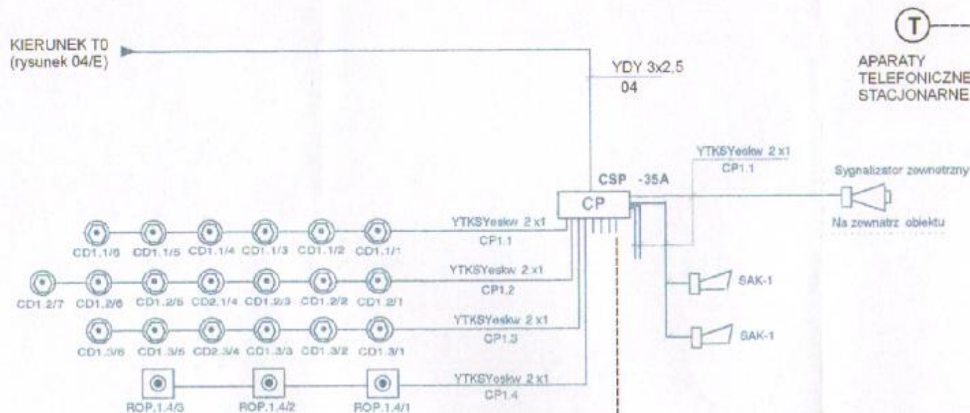
Przykładowe rozwiązanie instalacji p.pożarowej
