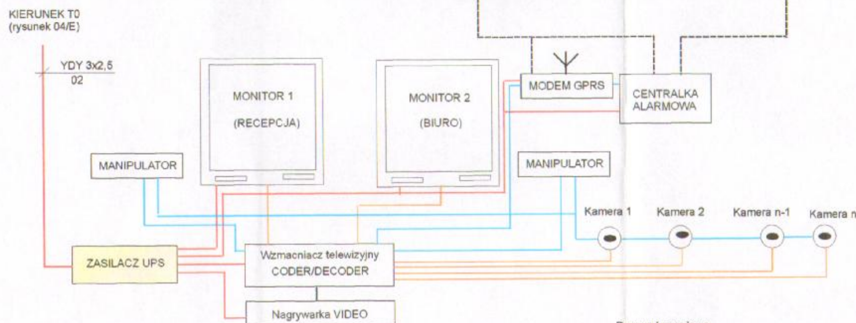
Przykładowe rozwiązanie instalacji monitoringu wizyjnego
