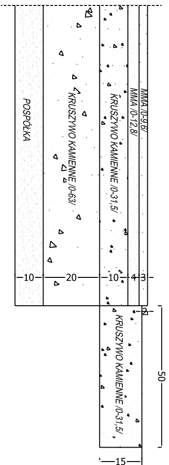
SCHEMAT KONSTRUKCJI JEZDNI WRAZ Z POBOCZEM
