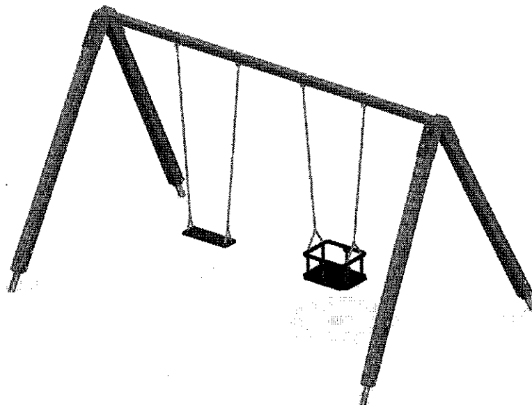
Rys. 2 Huśtawka łańcuchowa podwójna
